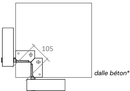
VUE D'ANCRAGE
