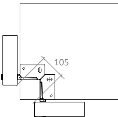
VUE D'ANCRAGE
