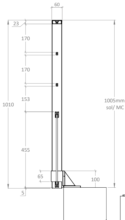
VUE DE COUPE
