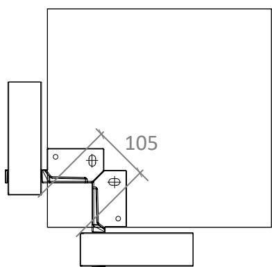
VUE D'ANCRAGE
