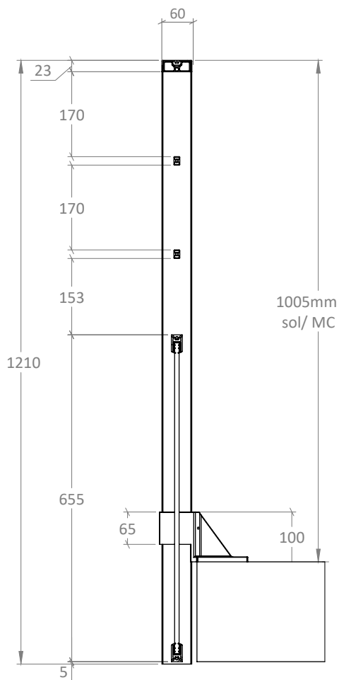
VUE DE COUPE
