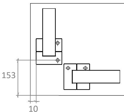
VUE D'ANCRAGE
