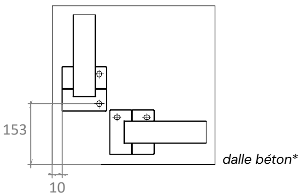
VUE D'ANCRAGE
